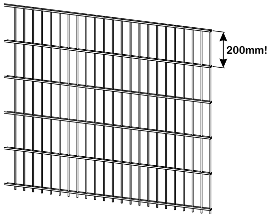
2x Doppelstabmatte Höhe gleich Zaunhöhe Länge variabel bis 2,5m
